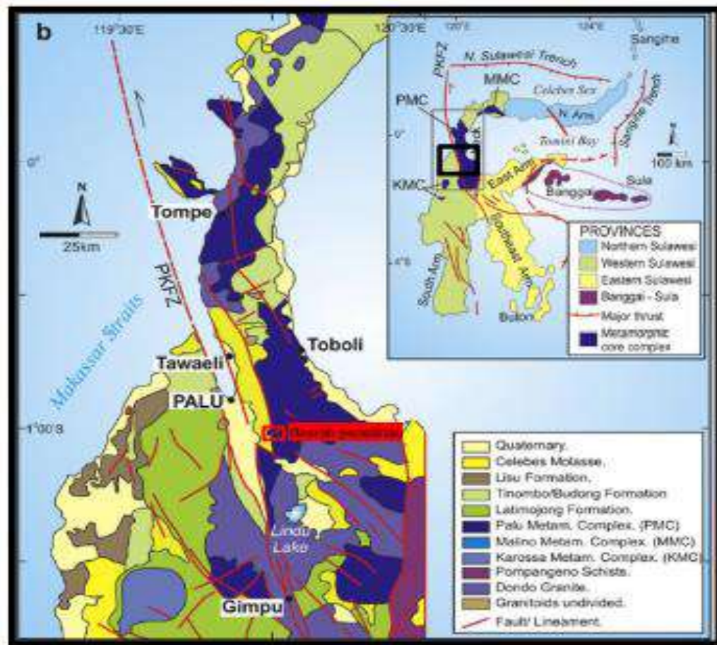
Gambar 2.2 Peta Geologi Provinsi Sulawesi Tengah
